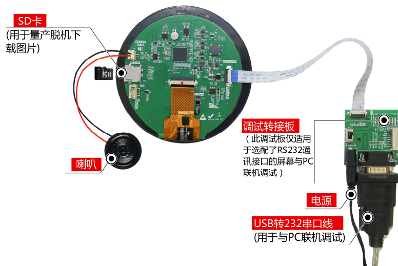
图 1-3 RS232 调试工具图
