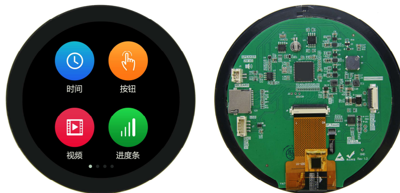
图 1-1 4.0 寸电容触摸参考图
